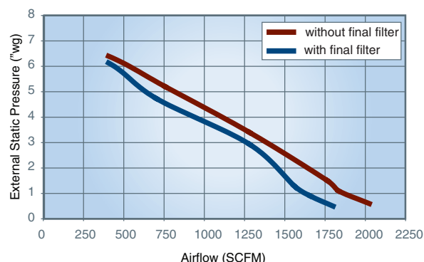
WSO 25-1* (3 HP)
